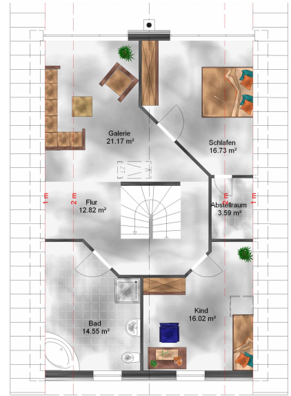
Obergeschoss
